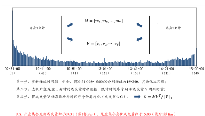
图33：成交重心的计算示意图
